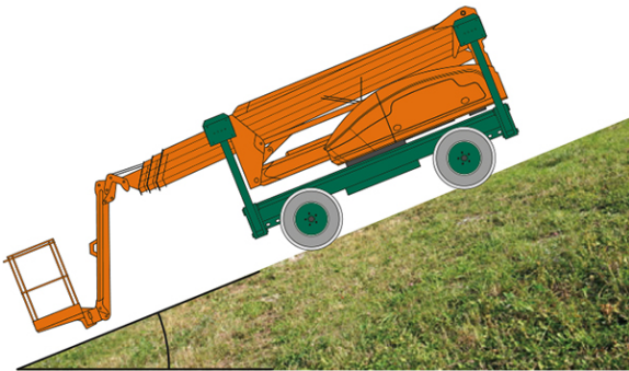
bis zu 40% oder 22° max. Steigfähigkeit
