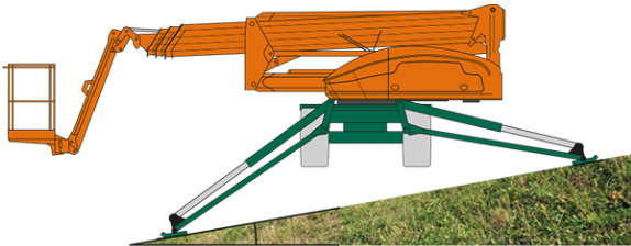
Ausgleich über Stützen max. 10°
